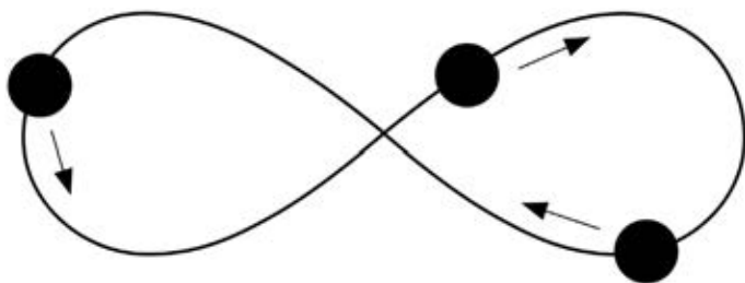
Órbita en forma de 8 de tres cuerpos.
